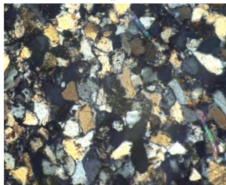
Рис. 7. Пісковик кварцовий з мусковітом та рудним мінералом (чорне): a – Ніколі II. 36 64; б – Ніколі X. 36 64.
