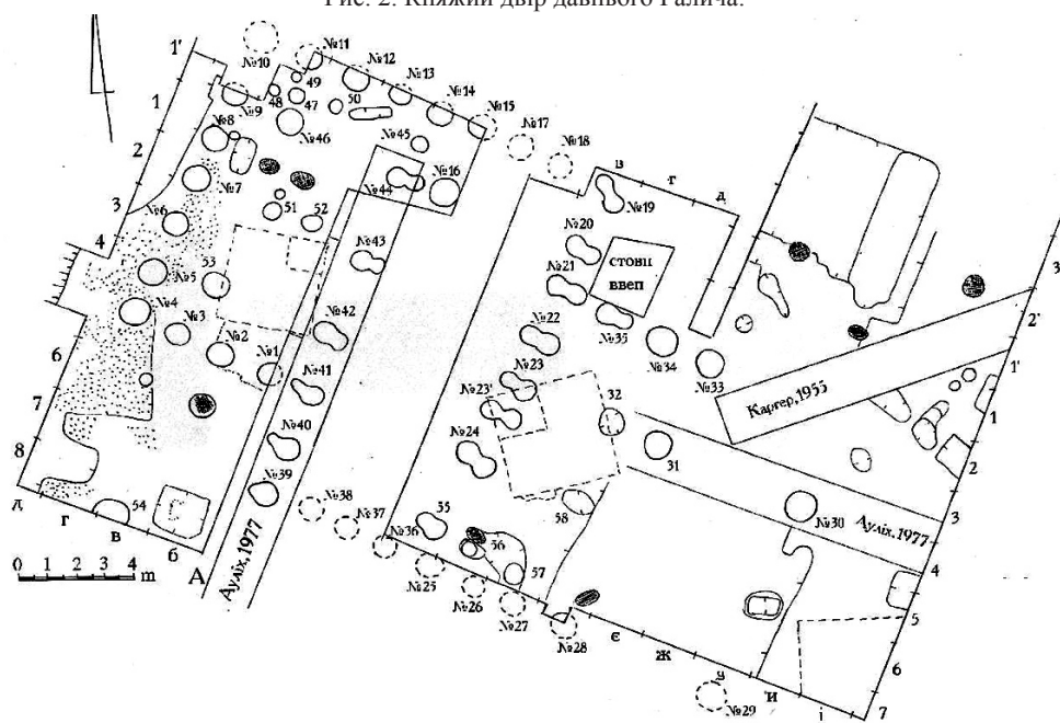
Рис. 3. Західний палацовий комплекс давнього Галича. Розкоп П. План.
